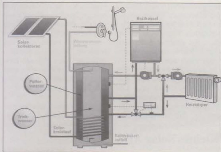
Schematische Darstellung einer Solaranlage
